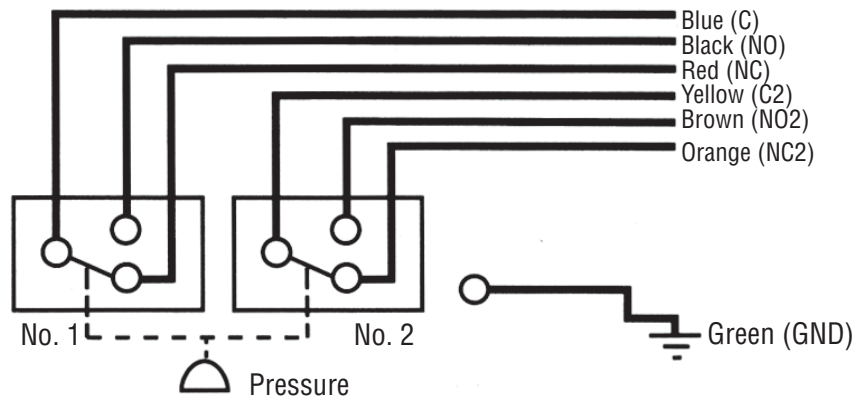
DPDT (2-SPDT)
